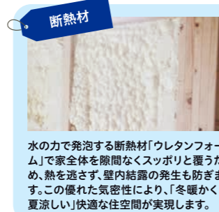
断熱材 水のかたまりで発泡する断熱材「ウレタンフォーム」で家全体を隙間なくスッポリと覆うため、熱を逃さず、壁内結露の発生も防ぎます。この優れた気密性により、「冬暖かく、夏涼しい」快適な住空間が実現します。
