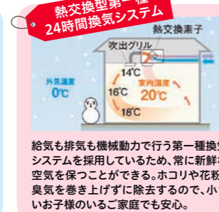
熱交換型第一種 24時間換気システム 給気も排気も機械動力で行う第一種換気システムを採用しているため、常に新鮮な空気を保つことができる。ホコリや花粉、臭気を巻き上げずに除去するので、小さいお子様のいるご家庭でも安心。
