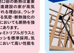
Kダンパー 「筋交いのみ」と「Kダンパー」を取り付けた家で震度7を再現した地震を合計10回連続させて実験しました。実験の結果、揺れ幅が最大76%低減され、ほぼ損傷がなく、繰り返しの揺れを抑える性能が高いことが証明されています。
